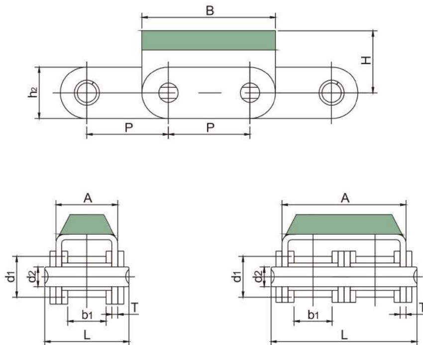
带D1部件 With D1 profile
